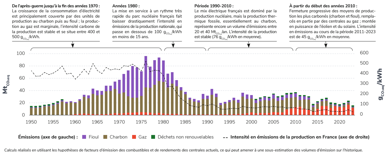
Figure 24 : Émissions directes de gaz à effet de serre liées à la production d'électricité en France et intensité en émissions de la production d'électricité française entre 1950 et 2023
