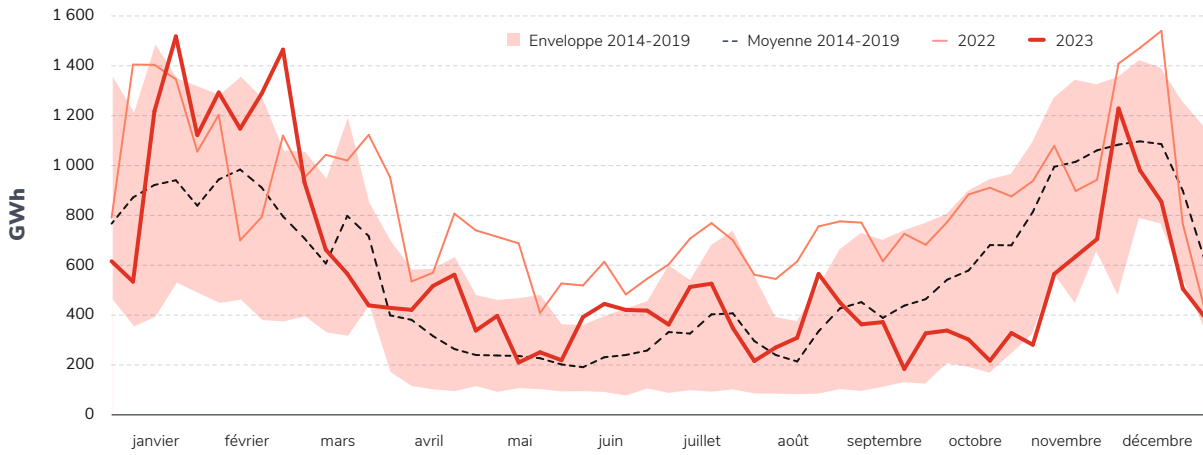
Figure 15 : Évolution de la production hebdomadaire des centrales au gaz au cours de l'année 2023 et comparaison avec les années précédentes
